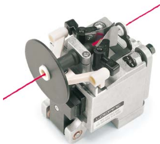
Keramikfederbremse
