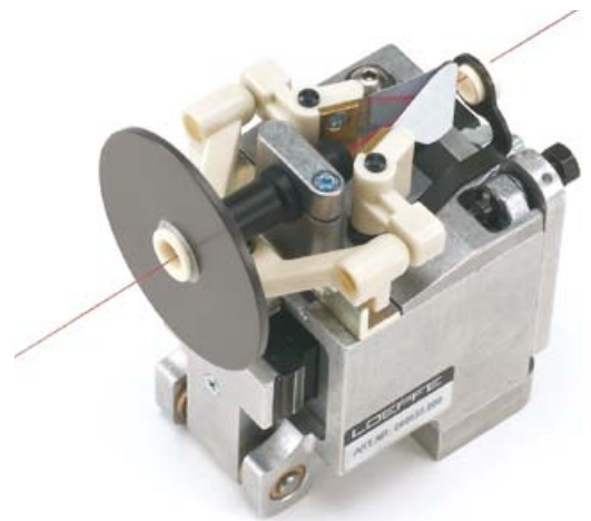
Chromfederbremse lang
