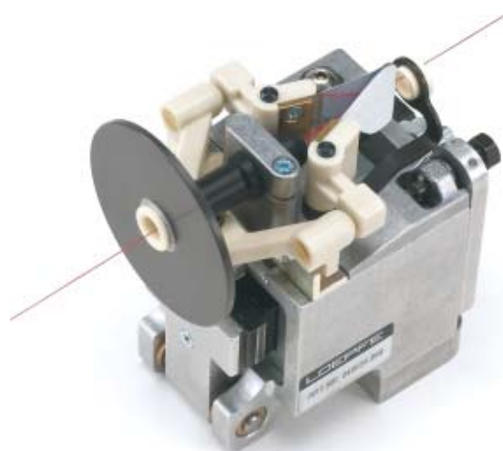
Freno de muelle de cromo largo
