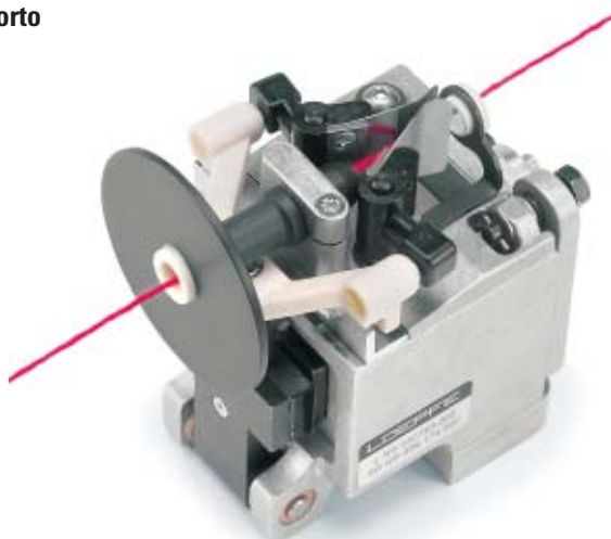
Freno de muelle de cerámica
